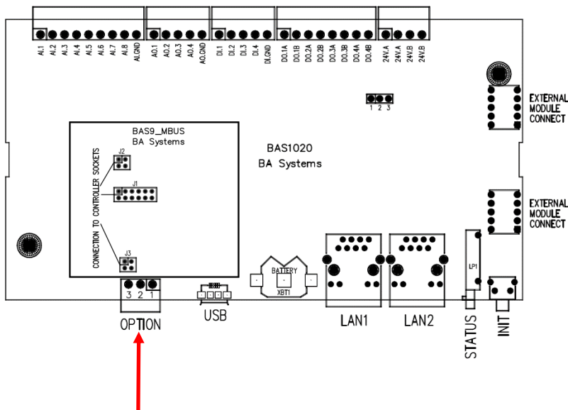
BAS1020 BAS9_MBUS module mount
